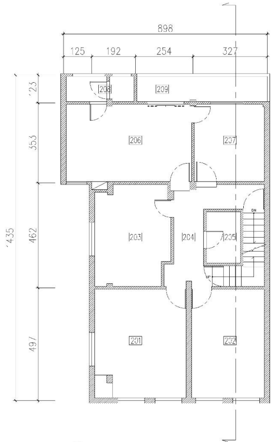
2 2樓平面圖 scale: 1/100 A2-52-1
