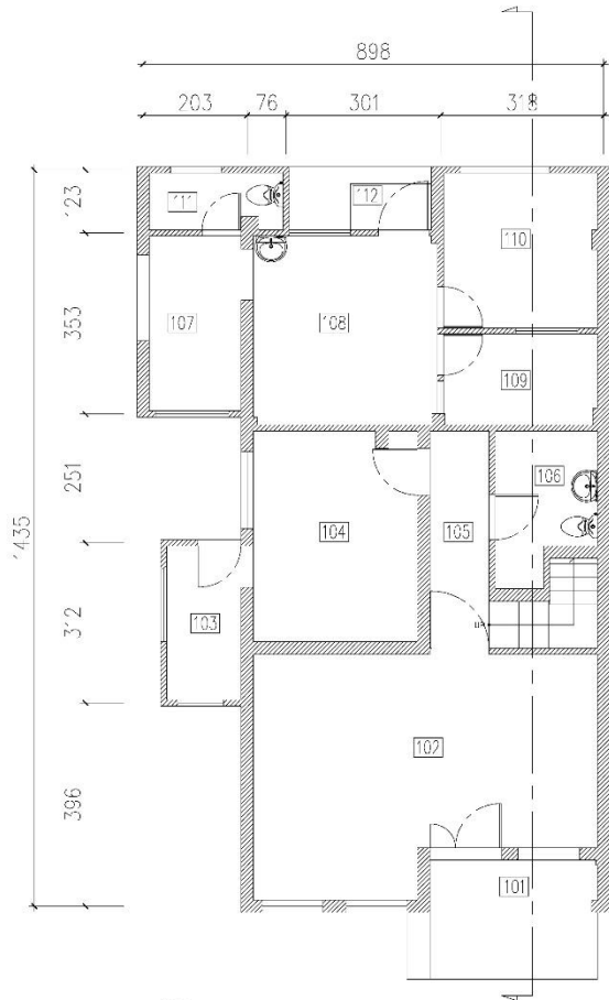
1 1樓平面圖 scale: 1/100 A2-52-1
