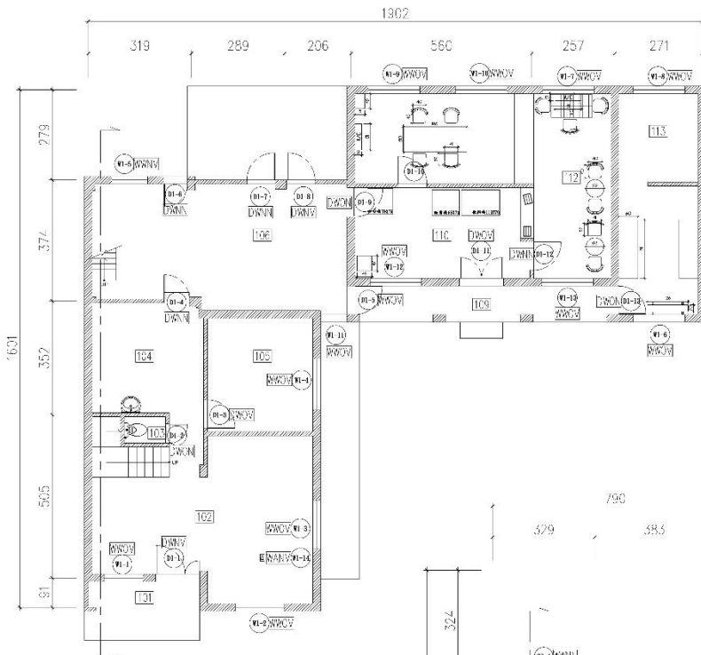
A2-53-1 一樓平面圖 scale: 1/100
