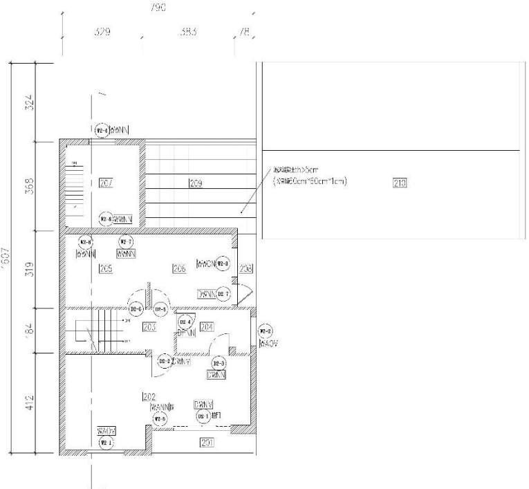
A2-53-2 二樓平面圖 scale: 1/100
